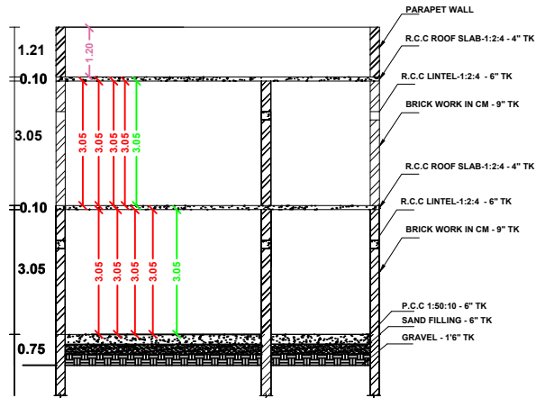
SECTION A-B
