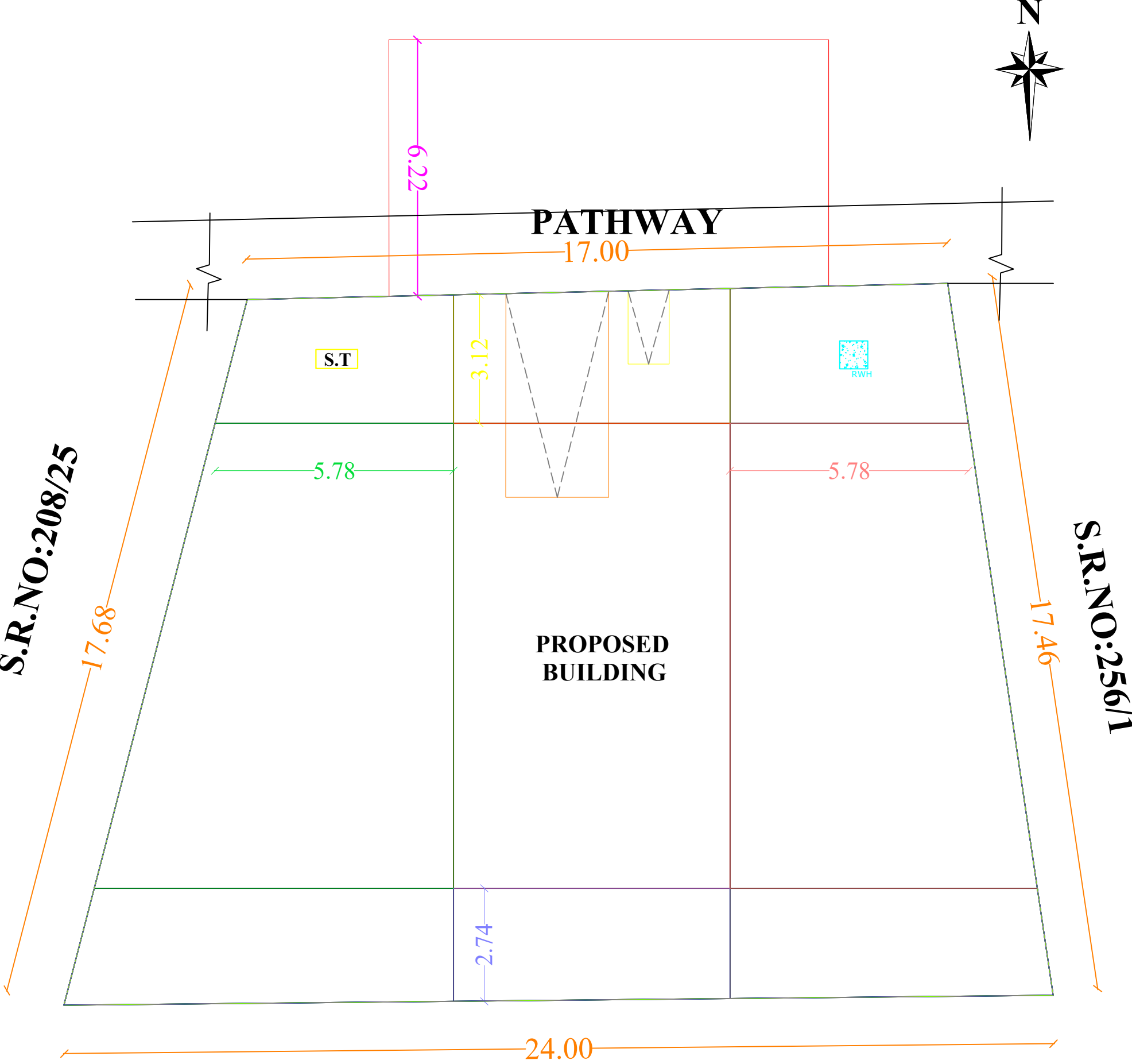
SITE PLAN:-
