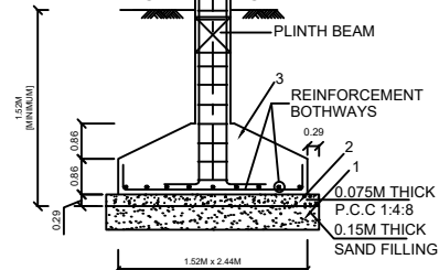
TYP. DET. COLUMN FOOTING
