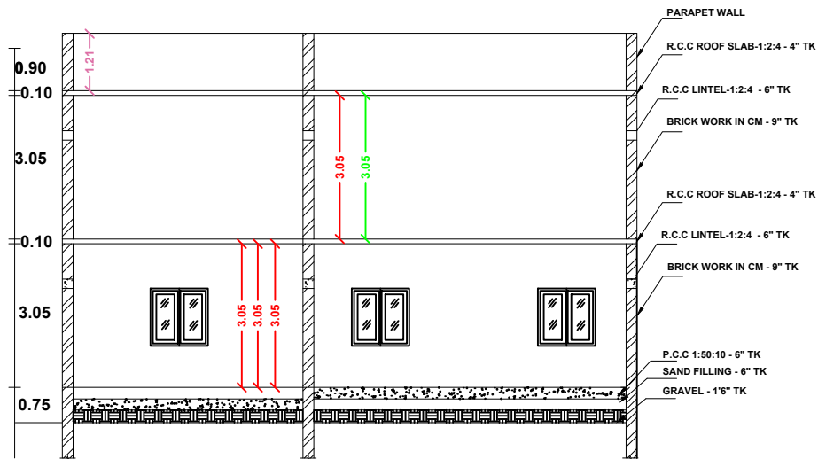
SECTION -AB
