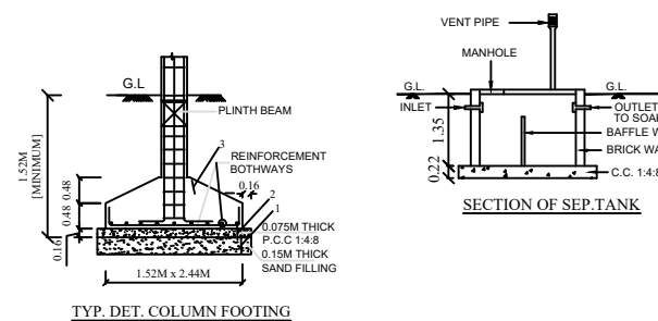
TYP. DET. COLUMN FOOTING
