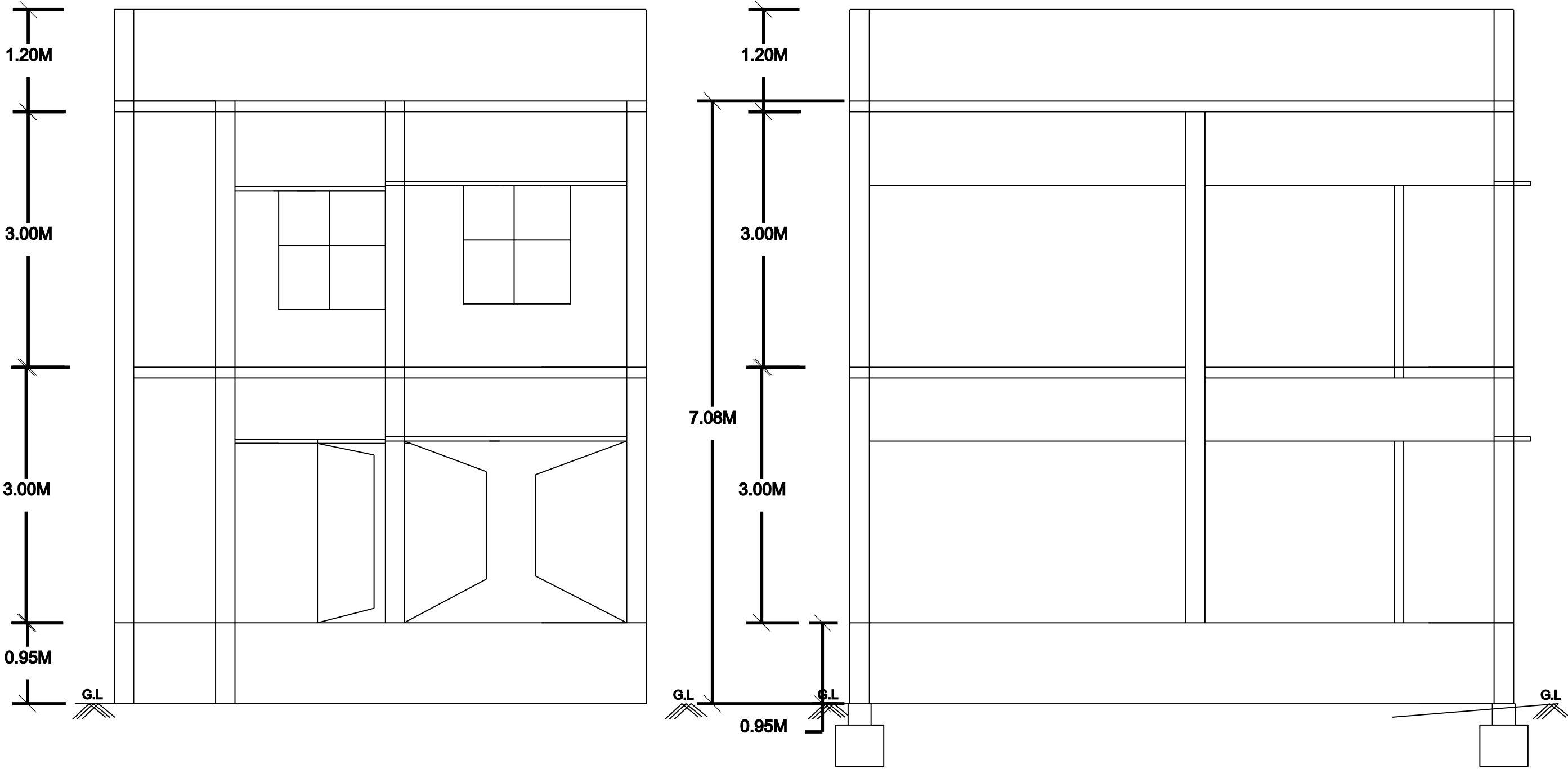
ELEVATION
