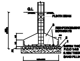
TYP. DET. COLUMN FOOTING
