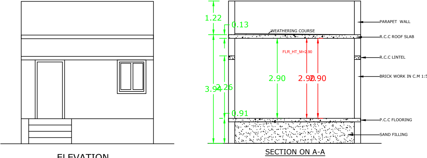
ELEVATION
