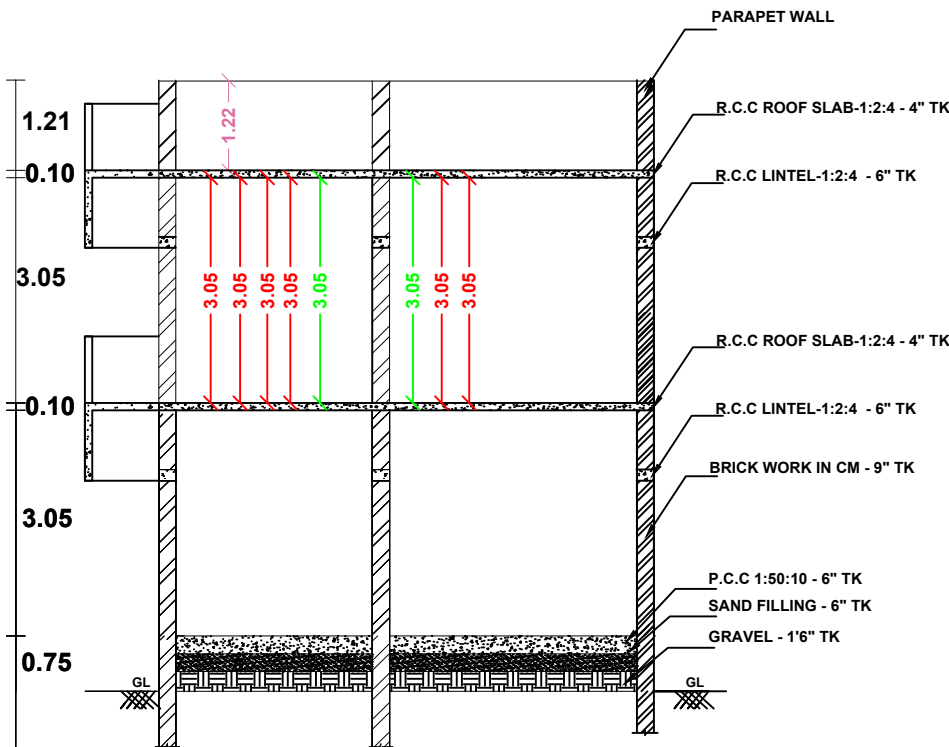
SECTION A-B
