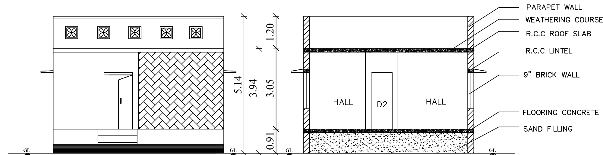
ELEVATION
