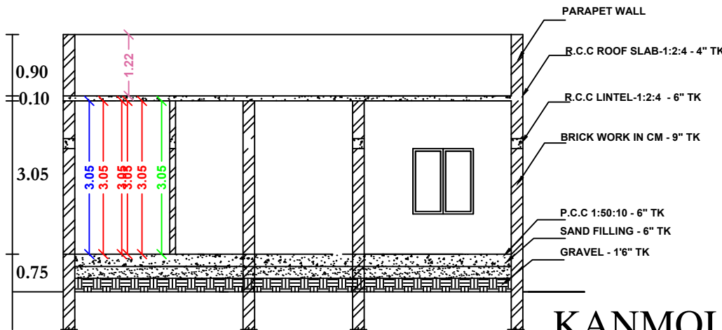
SECTION -AB
