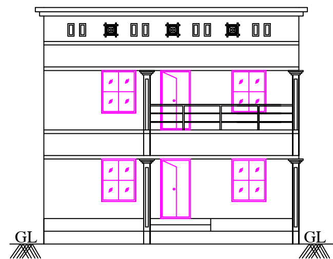
ELEVATION
