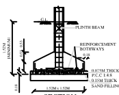
1.52M x 1.52M SECTION
