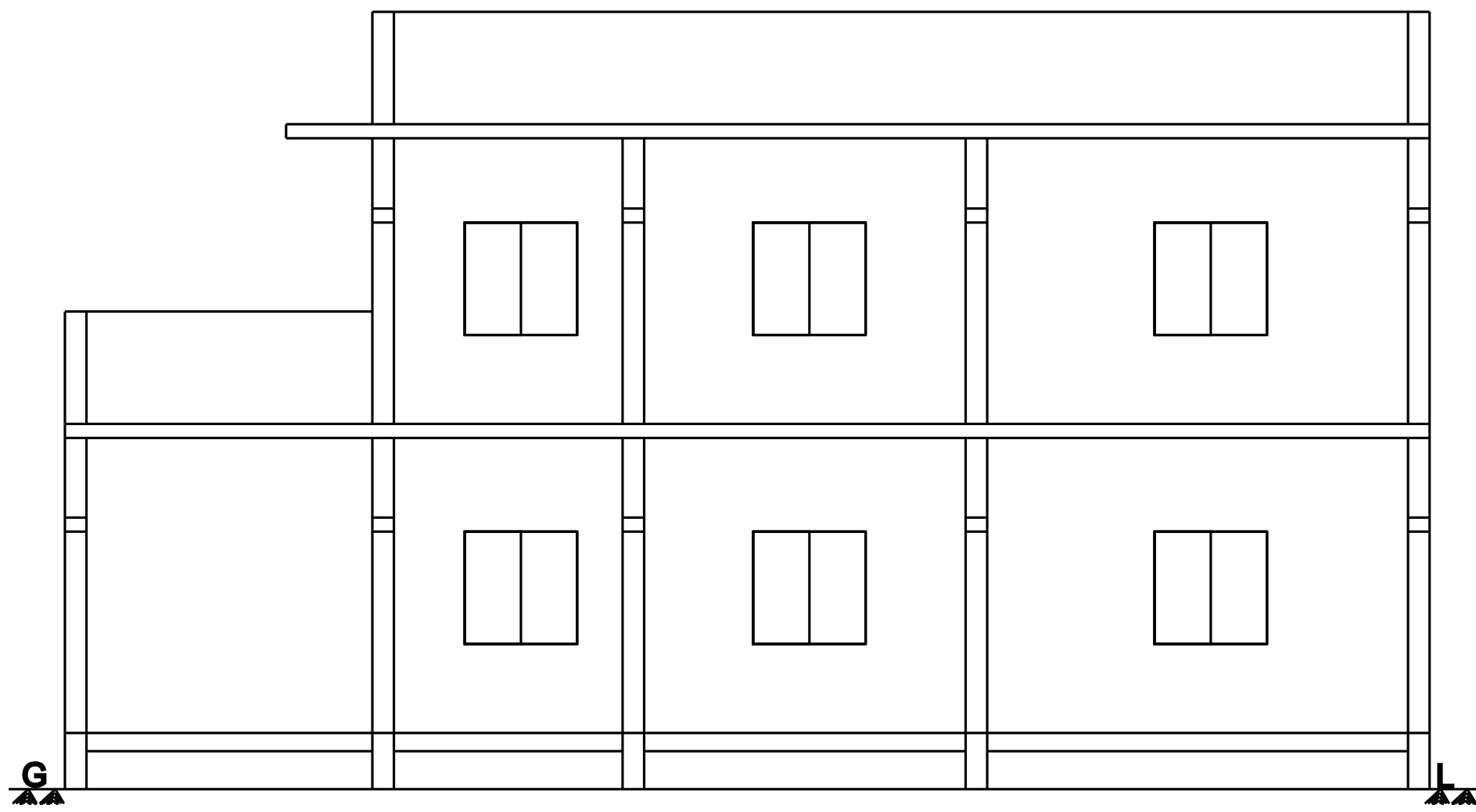
SECTION ON'RP'
