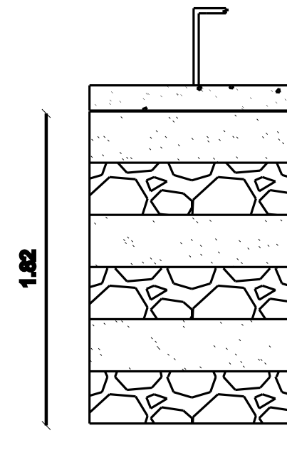
SECTION ON R.W.PITS
