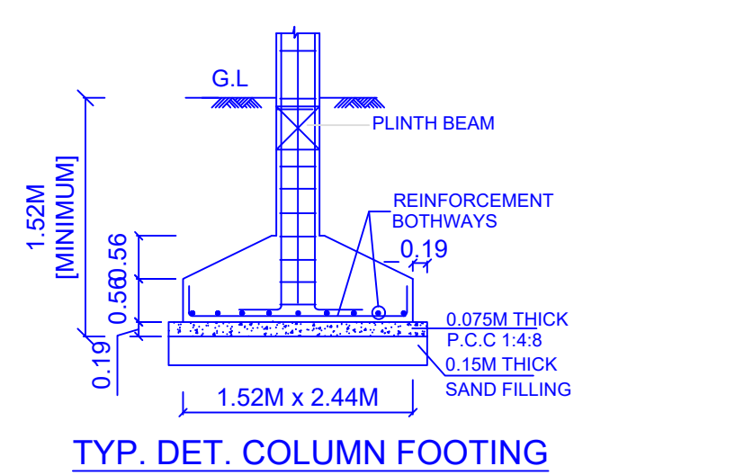
TYP. DET. COLUMN FOOTING
