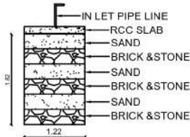
SECTION ON R.W.PITS
