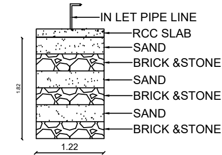
SECTION ON R.W.PITS
