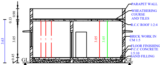
SECTION R-C
