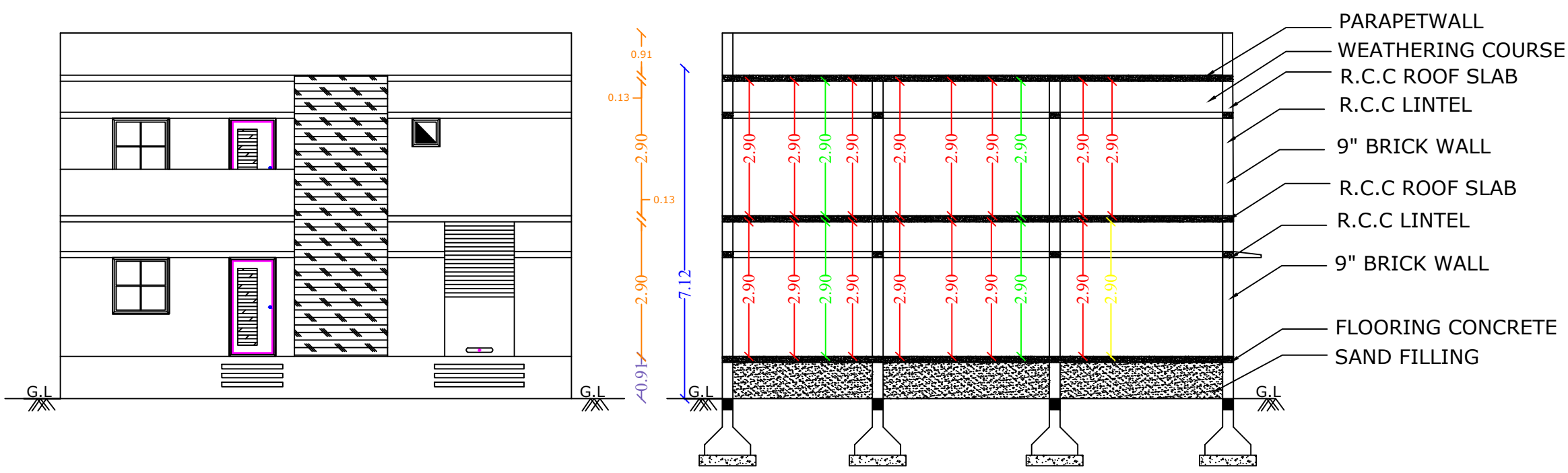
SECTION A-A'
