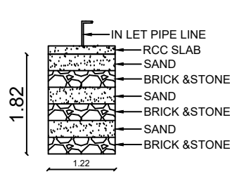
SECTION ON R.W.PITS
