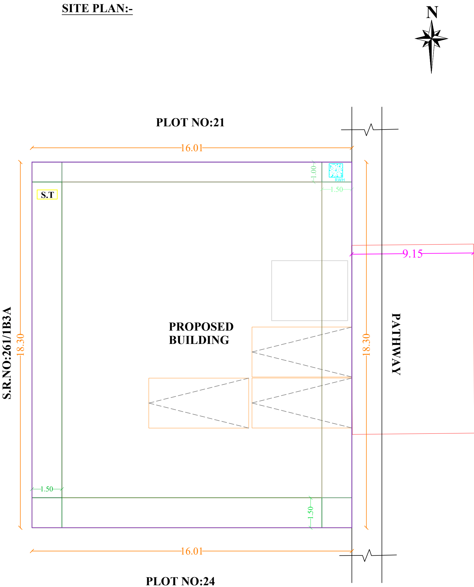
SITE PLAN:-
