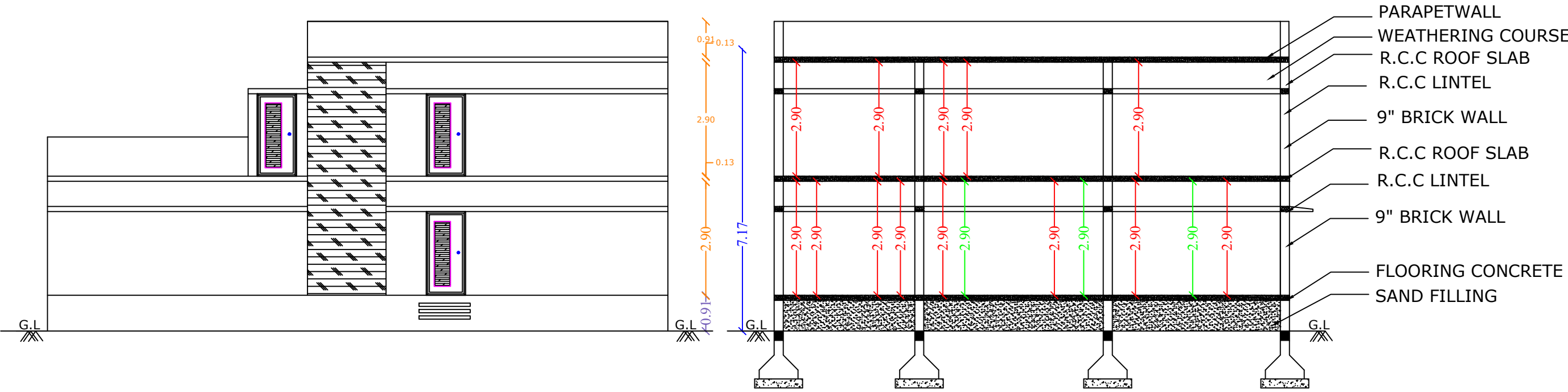
SECTION A-A'
