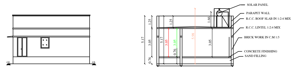
ELEVATION
