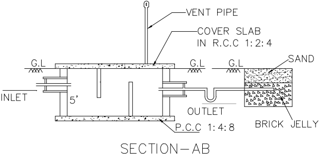
SECTION - AB
