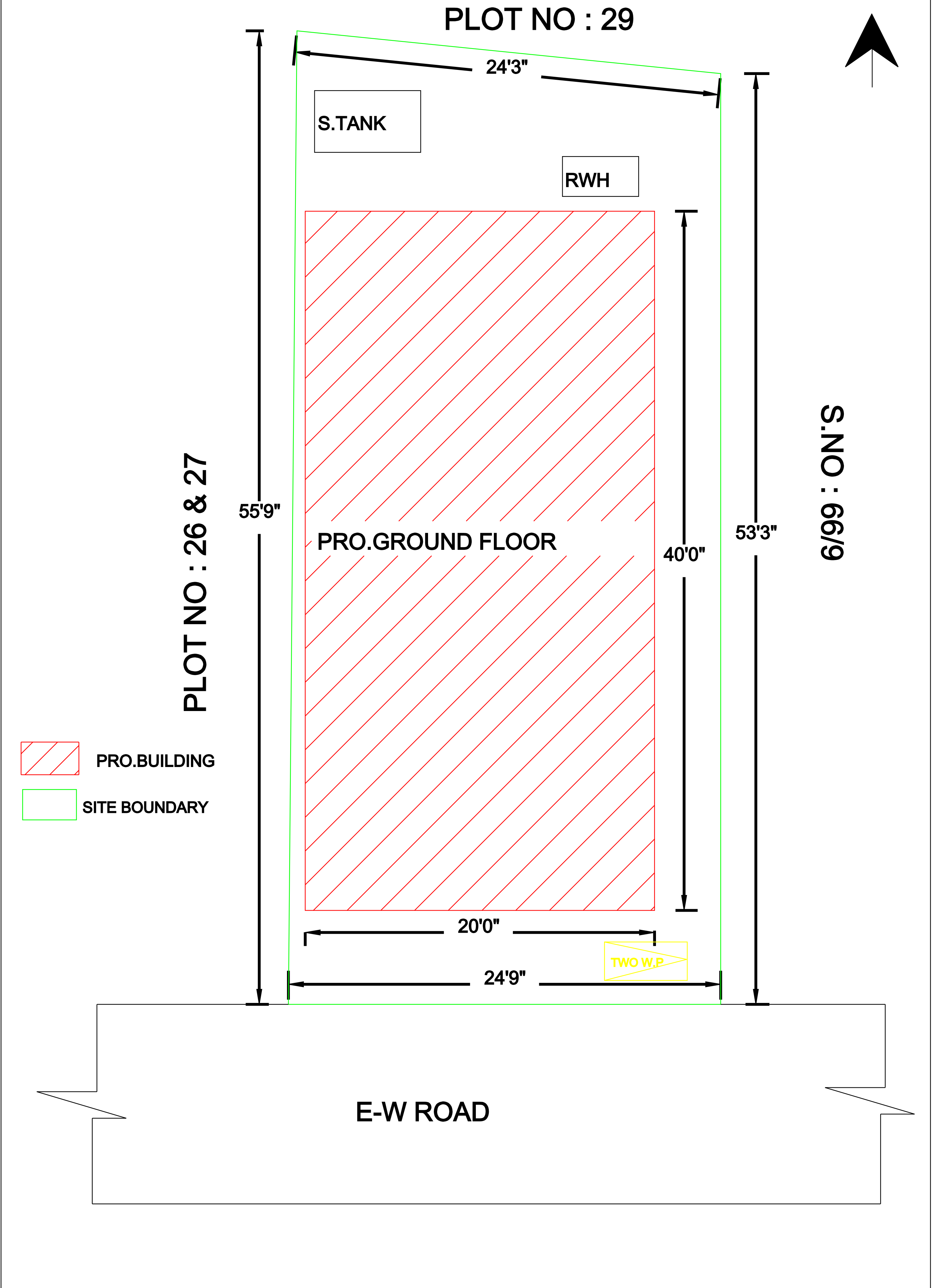
SITE PLAN :
