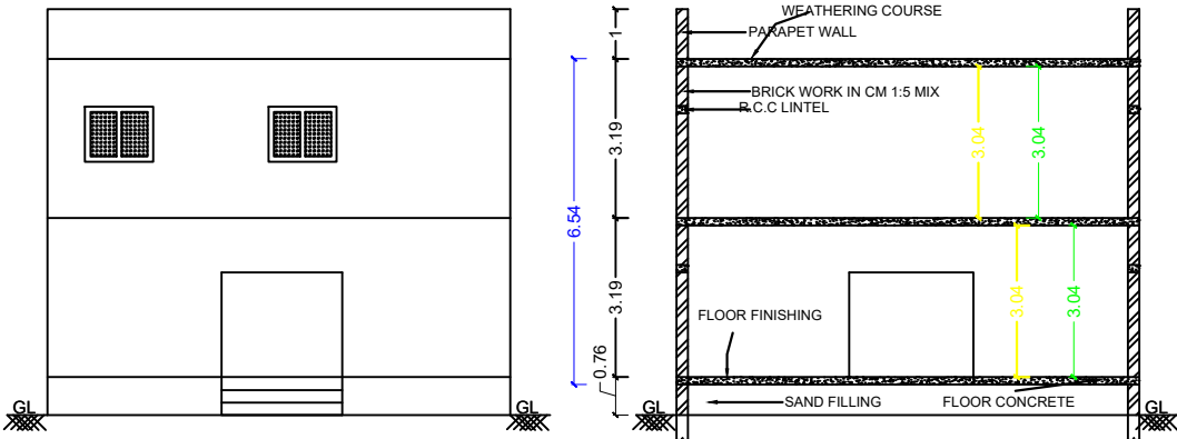
ELEVATION
