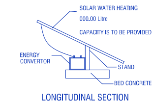
LONGITUDINAL SECTION
