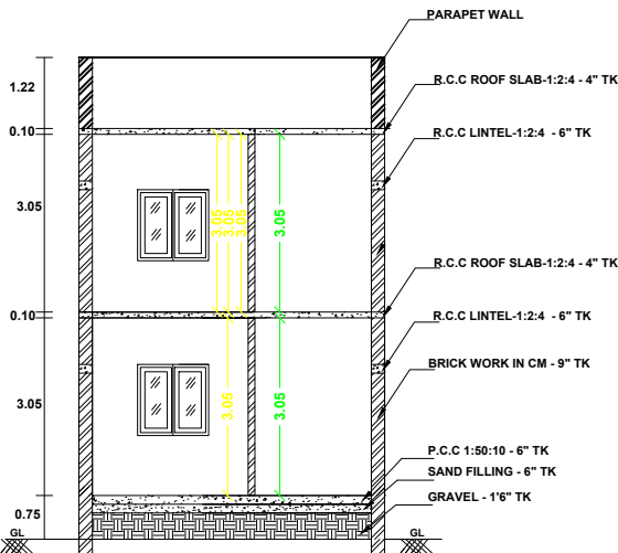
SECTION -AB
