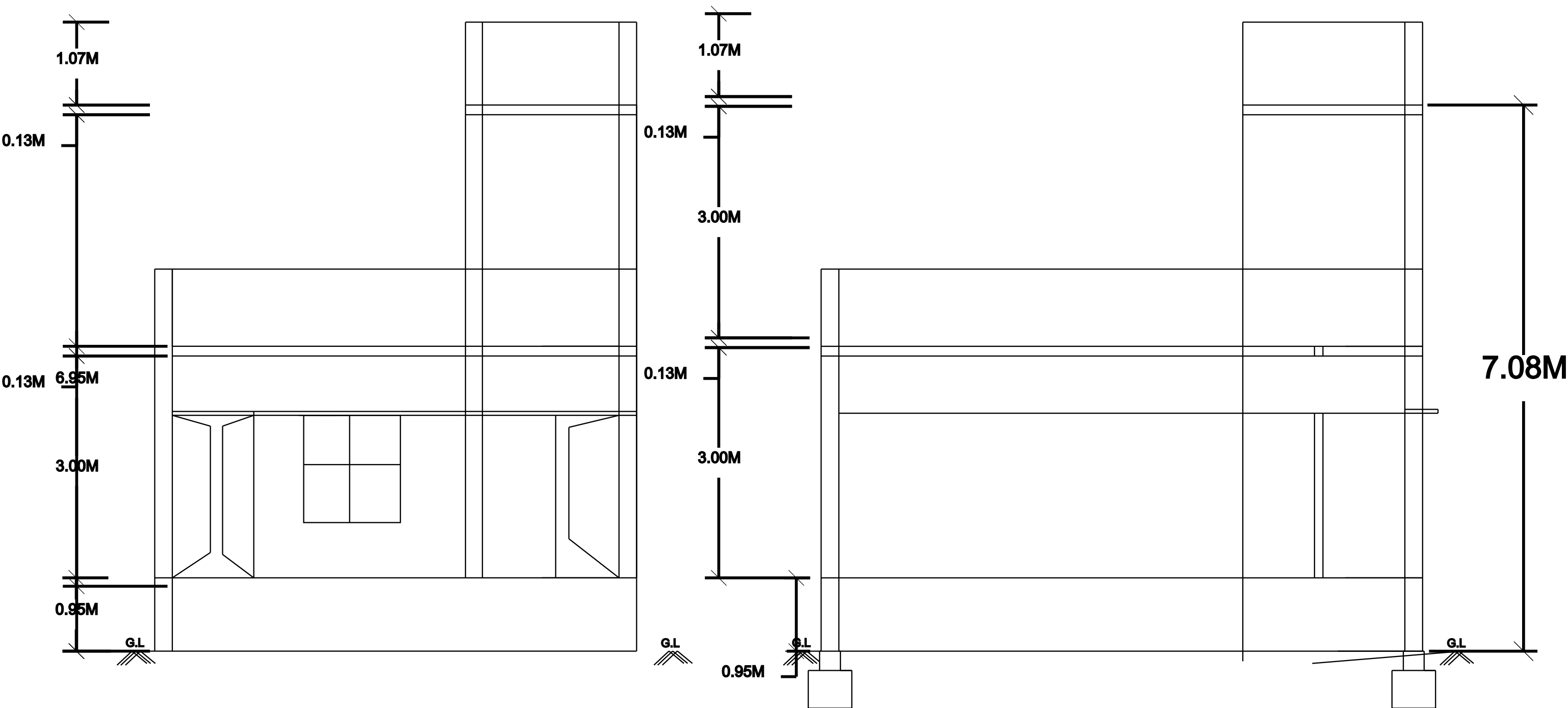
ELEVATION
