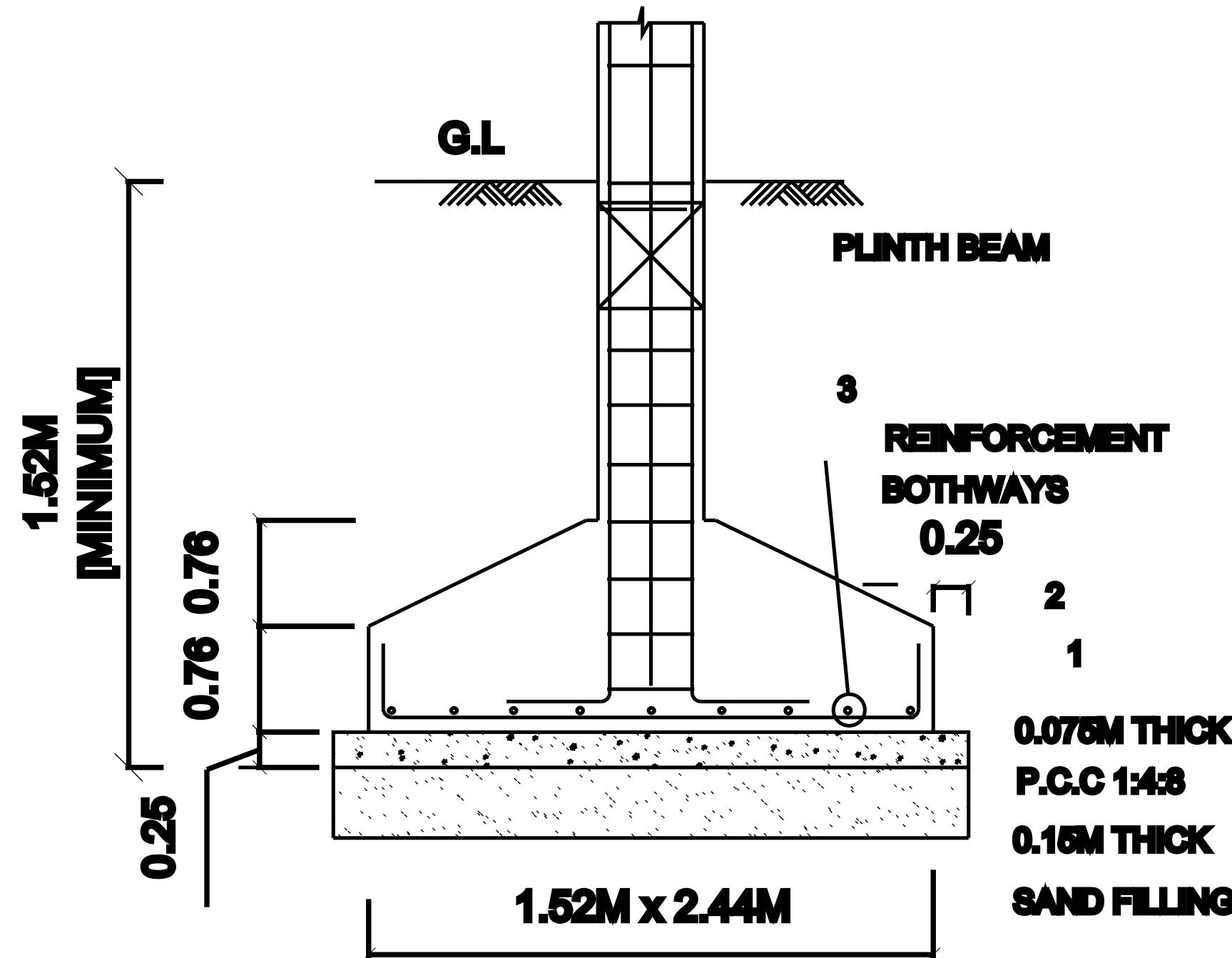
TYP. DET. COLUMN FOOTING
