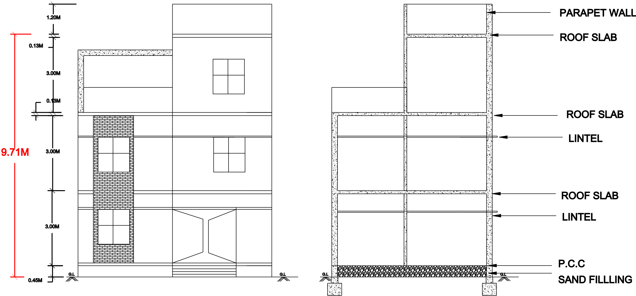
ELEVATION
