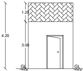
ELEVATION
