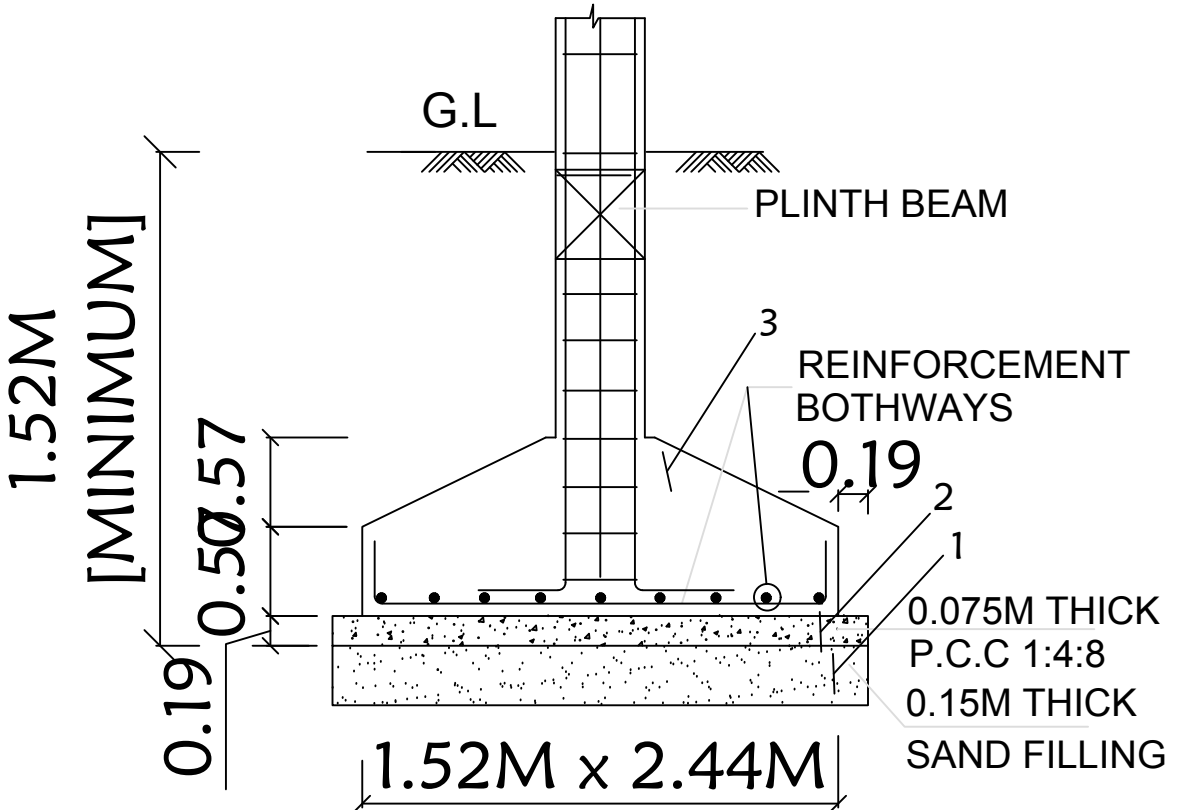
TYP. DET. COLUMN FOOTING
