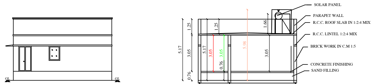
ELEVATION
