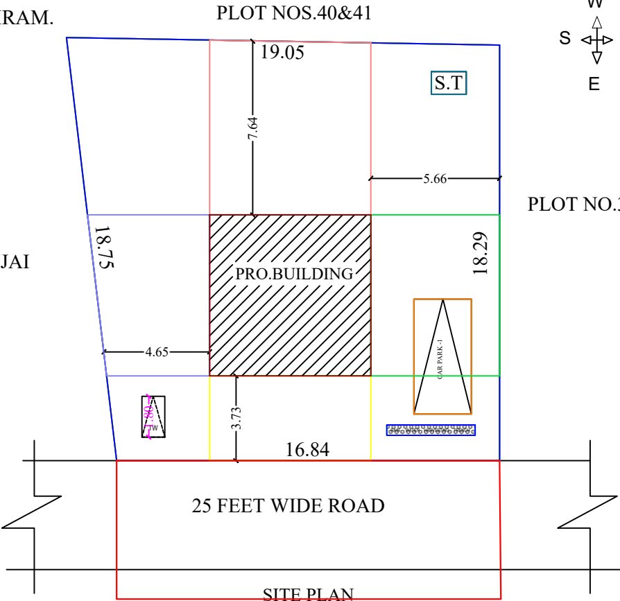
SCALE:1:200
