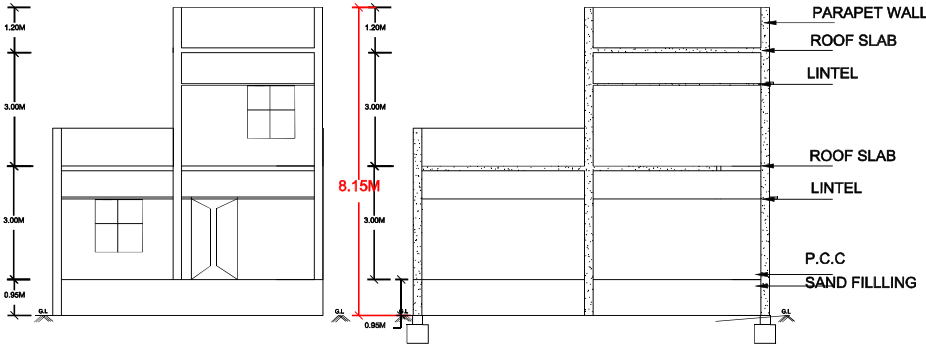
ELEVATION
