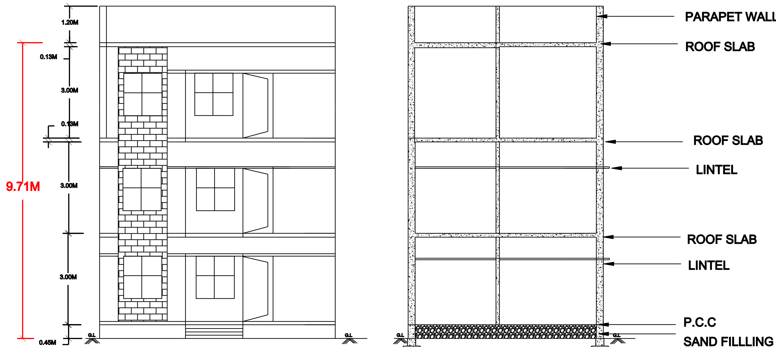
ELEVATION
