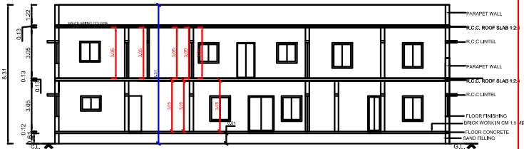
SECTION A-A 1
