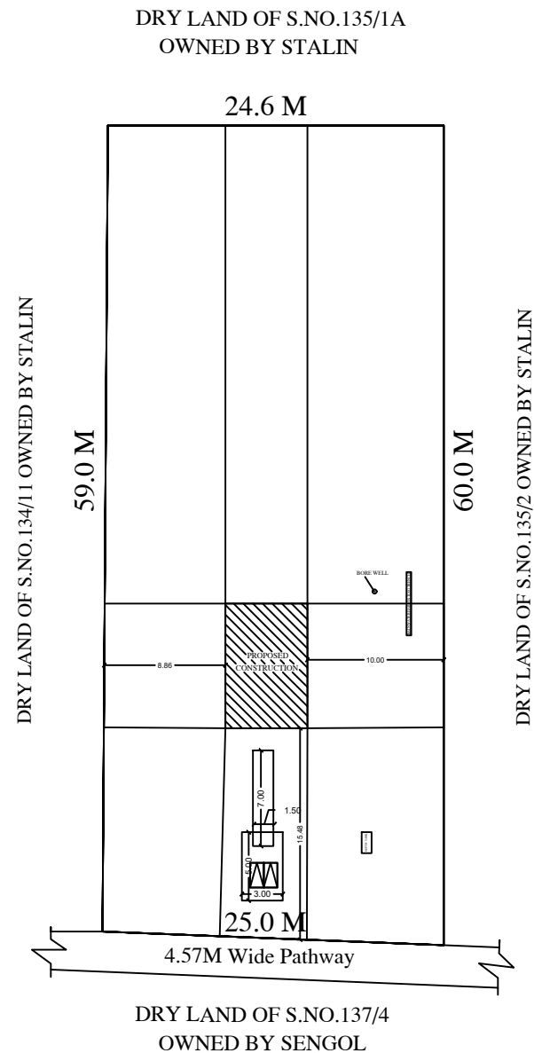
SITE PLAN(N.T.S)
