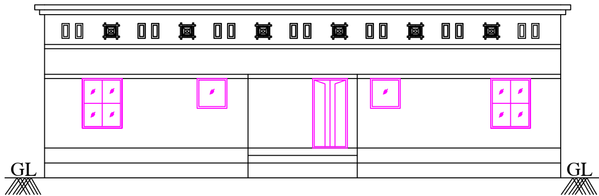
ELEVATION
