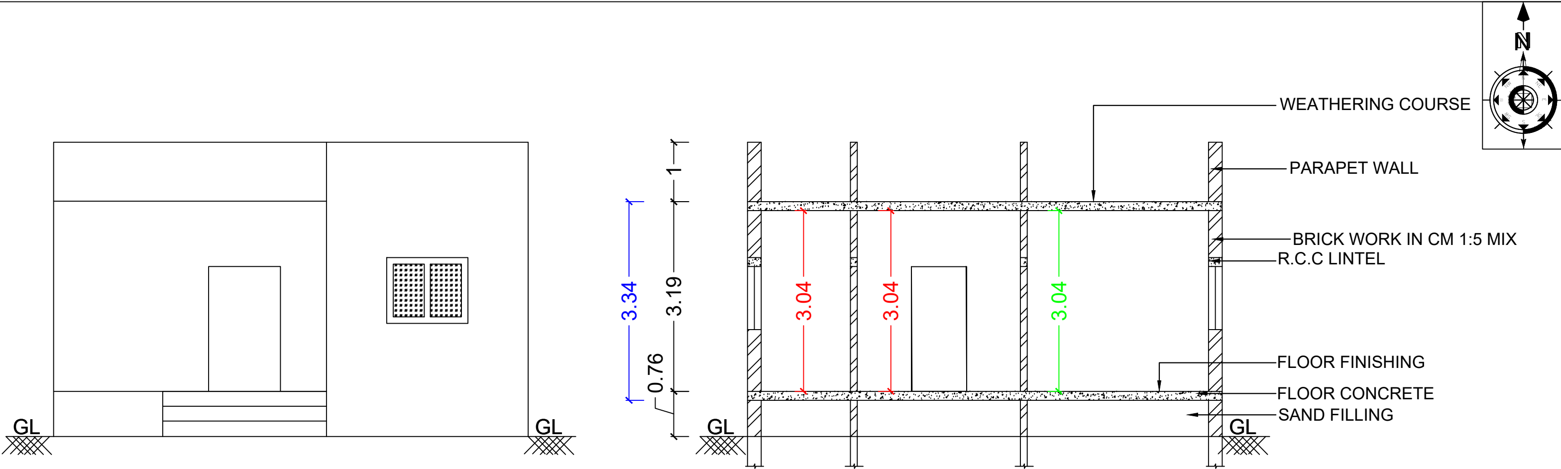
ELEVATION
