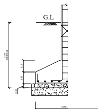
TYP. DET. COLUMN FOOTING
