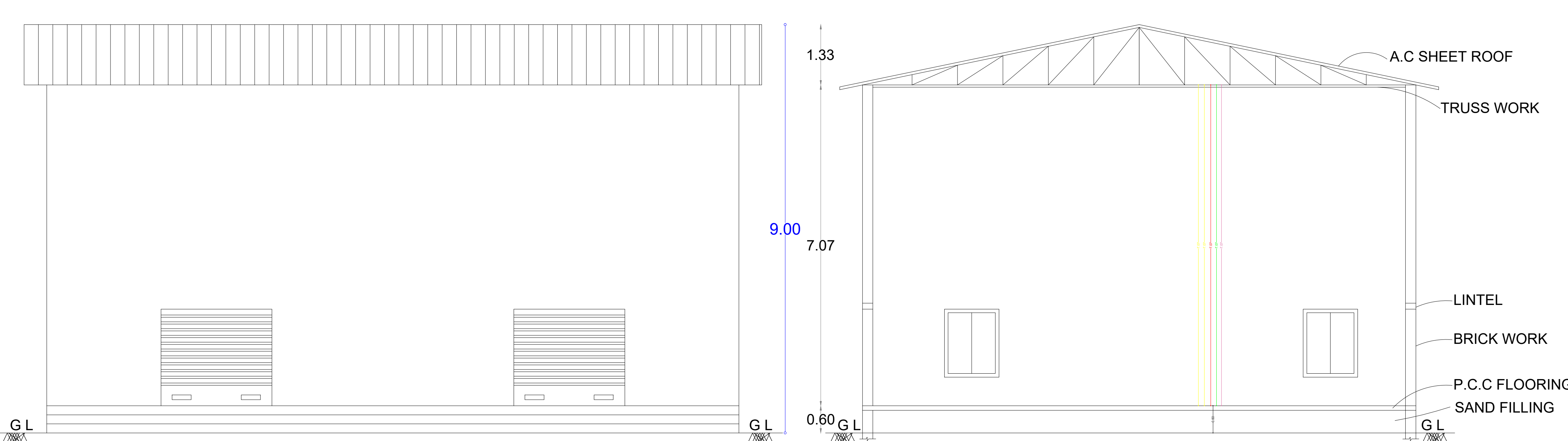
ELEVATION
