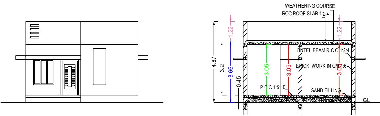
ELEVATION
