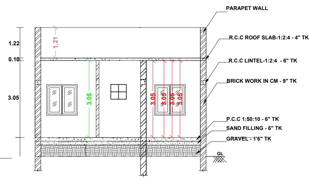
SECTION -AB
