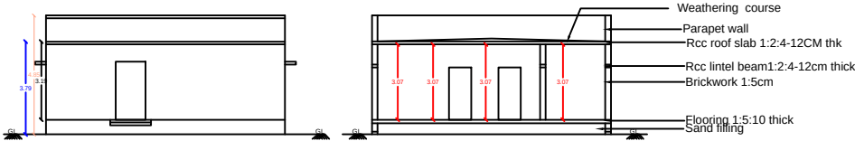
ELEVATION
