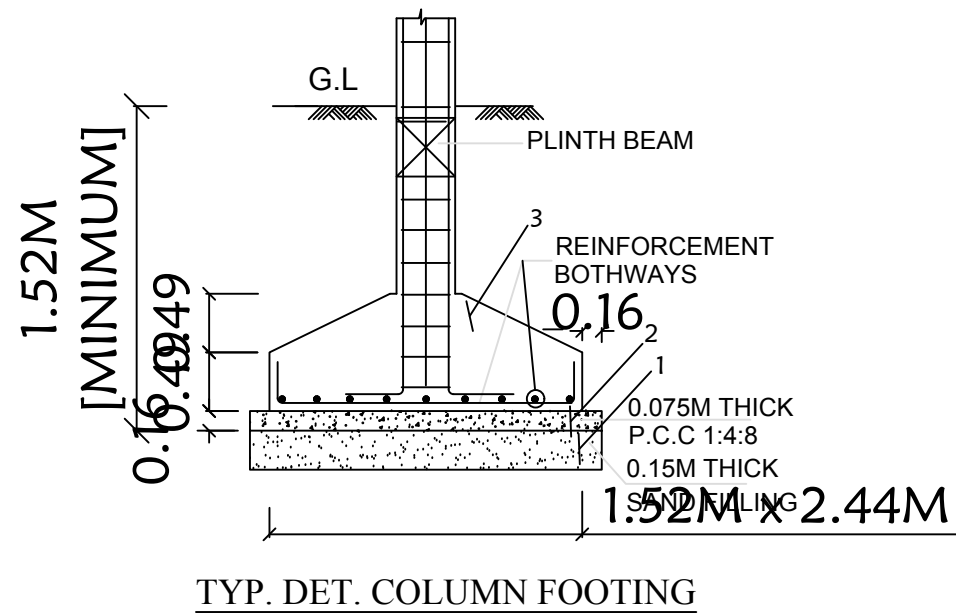
TYP. DET. COLUMN FOOTING
