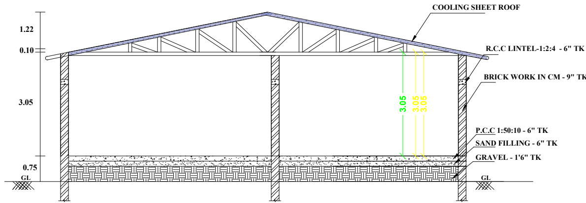
SECTION -AB
