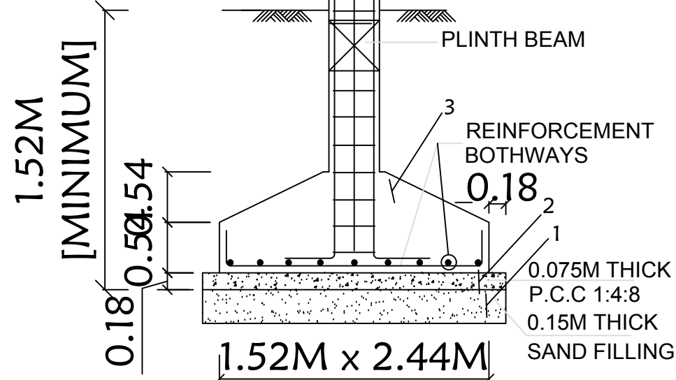
TYP. DET. COLUMN FOOTING
