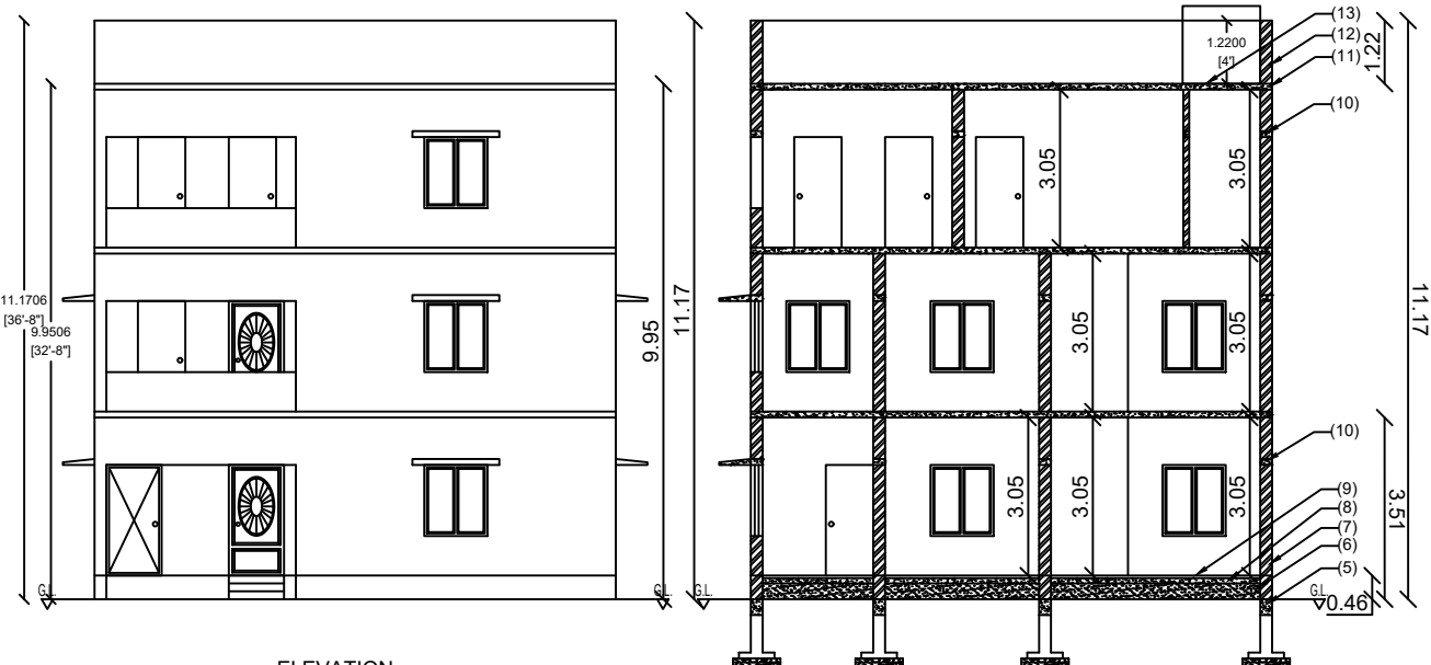
ELEVATION
