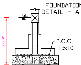
TYP. DET. COLUMN FOOTING
